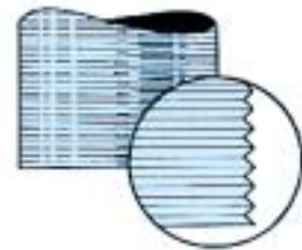
Punzón rectificado cilíndricamente. Aumento del riesgo de desconches, melladuras y desprendimientos.
