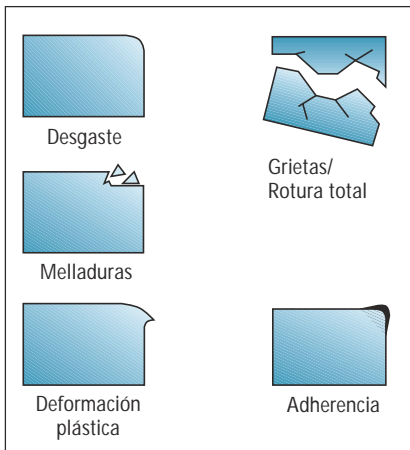
Fig. 2. Mecanismos de fallo más frecuentes en aplicaciones de trabajo en frío.
