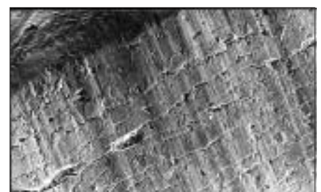
Fig. 6. Fotografía SEM de un punzón realizado con material D2 fuera de servicio a causa del desgaste adhesivo (material de trabajo, acero inoxidable austenítico).
