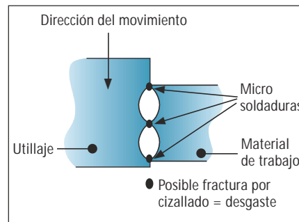
Fig. 4. Representación esquemática de desgaste adhesivo.
