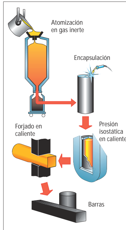
Fig. 8. Representación esquemática del proceso pulvimetalúrgico (PM) para la fabricación de acero.
