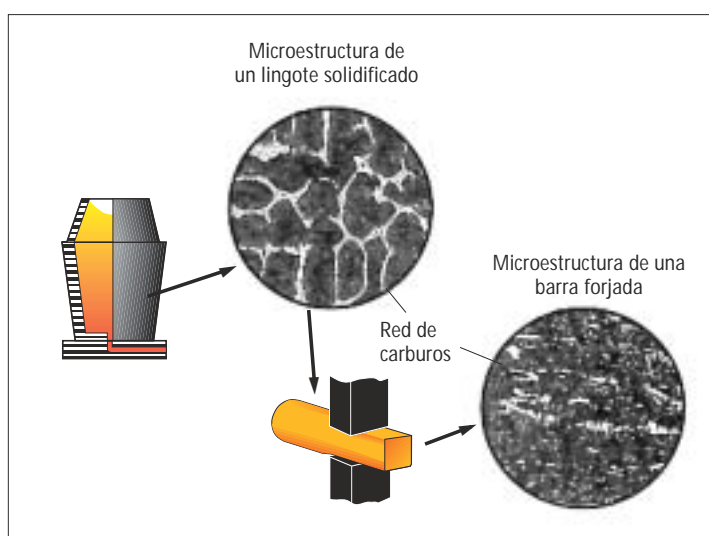
Fig. 7. Rotura de la red de carburos durante la operación de forjado en caliente de lingotes de acero.
