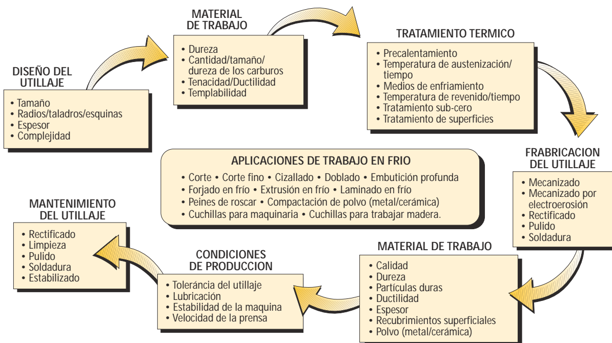
Fig. 1. Factores que influyen la vida del utillaje en aplicaciones de trabajo en frío.
