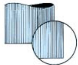
Punzón rectificado longitudinalmente. La suave penetración y acción de arranque aumenta la vida del punzón.
